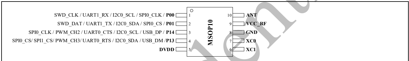
图 4-2 MSOP10 引脚图
