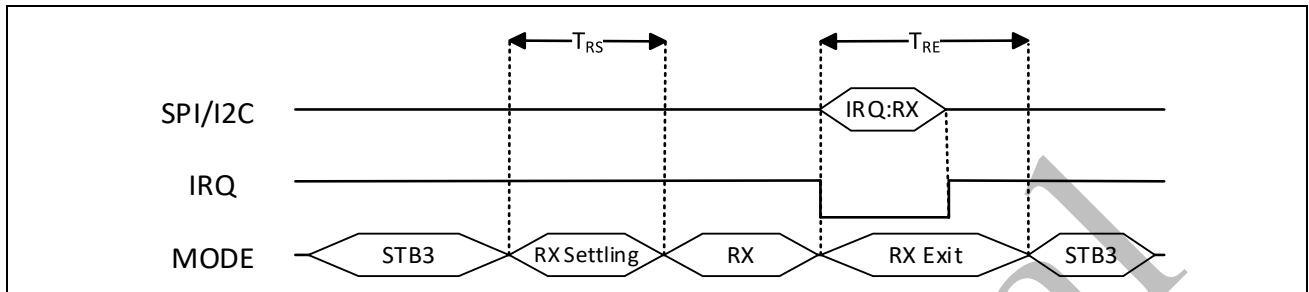
图 6-4 单包接收时序图
