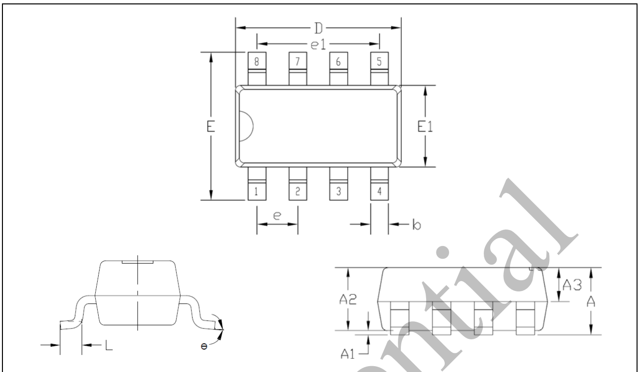
图 12-2 SOT23-8 封装图
