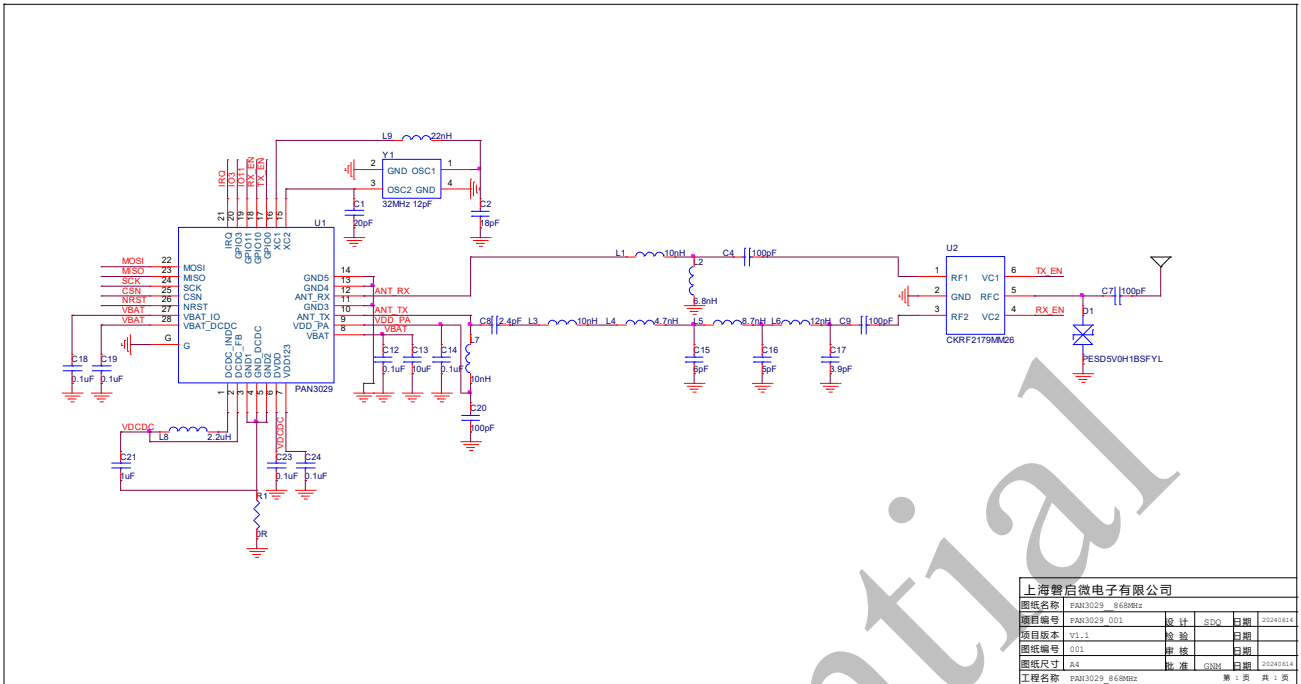
图 13-5 868MHz 参考原理图
