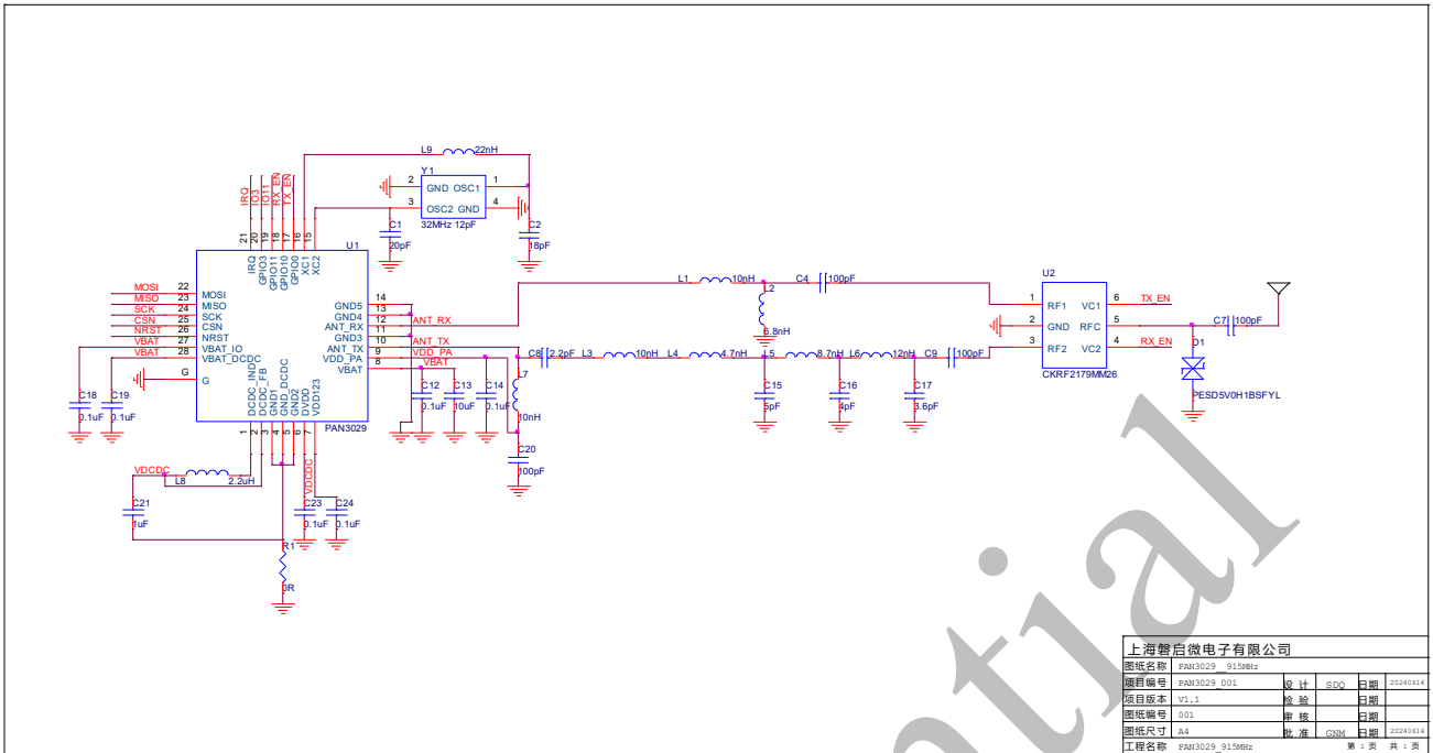
图 13-7 915MHz 参考原理图
