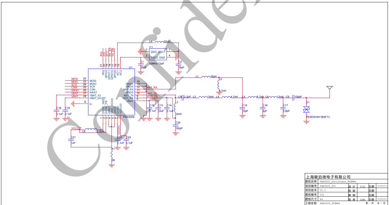
图 13-6 Switchless 868MHz 参考原理图
